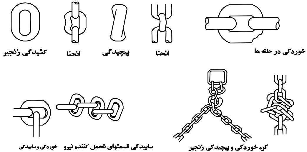
شکل شماره (۶-۲۲): نمونه‌هایی از زنجیرهای مستعمل
