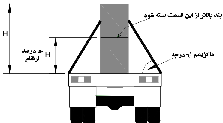
شکل شماره (۶-۱۳): نحوه بستن بندها برای ایجاد پایداری بار
